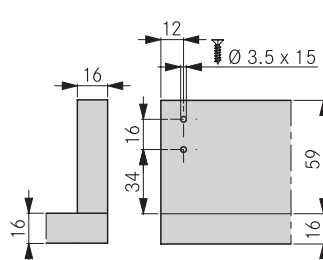
Схема за дупчене на гръб
