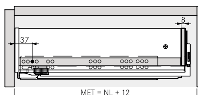
Минимална дълбочина за вътрешно чекмедже
