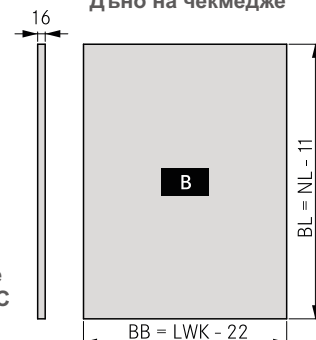
Дъно на чекмедже
