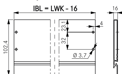
Схема за дупчене на челен панел
