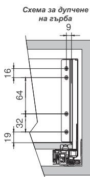
Гръб с дебелина 16 мм
