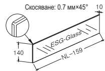
Стъклена страница 10 мм
