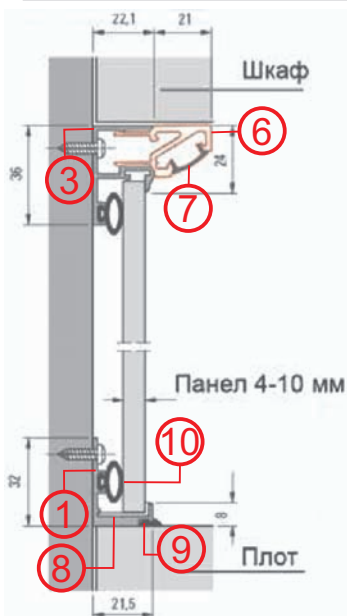
Система ТЕСНИ профили с монтиран профил и капачка за LED осветление
