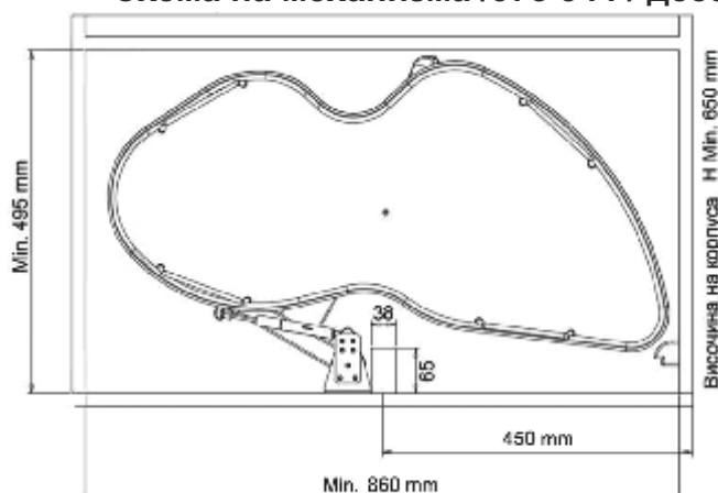
Схема на механизма /378 544 / десен
