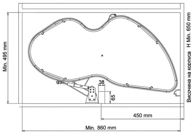
Схема на механизма /337 933 /
